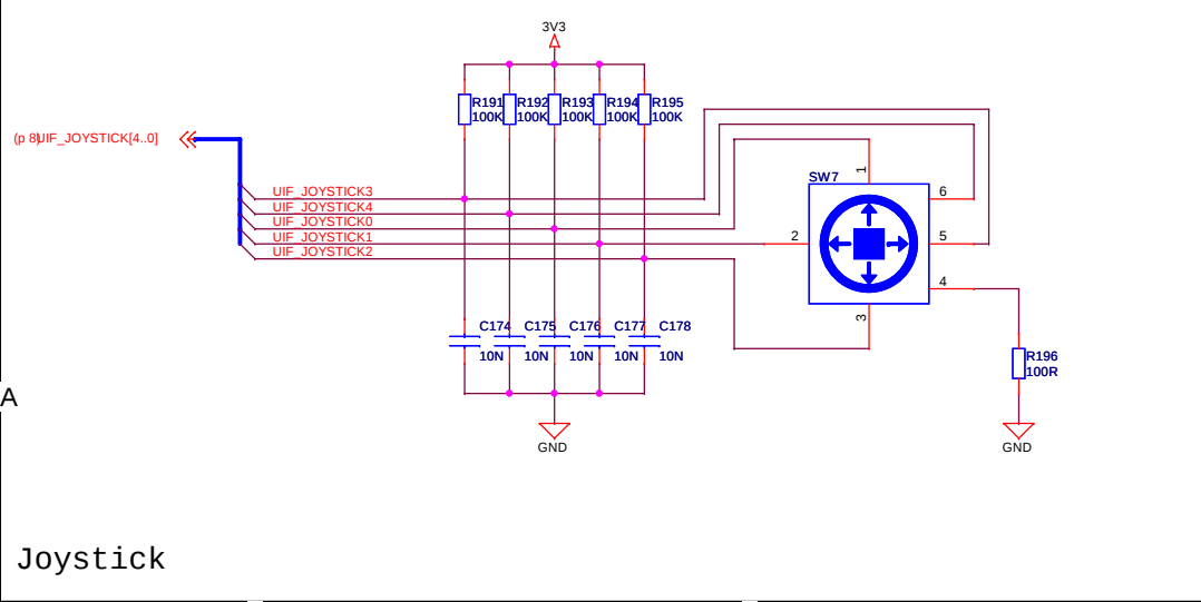
Joystick
